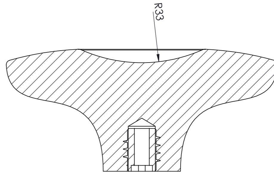
SECTION G-G SCALE 2 : 1
