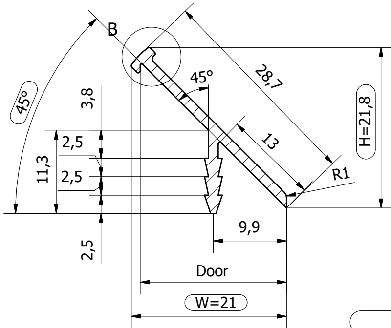
A-A ( 2/1 ) SECTION
