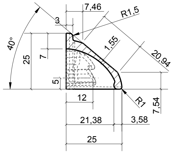
SEZIONE AA-AA
