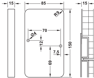
Montage: Griff einseitig
