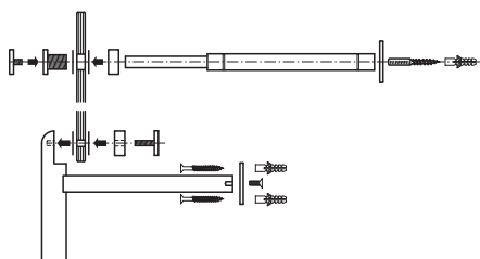
Montage mit Glasplatte
