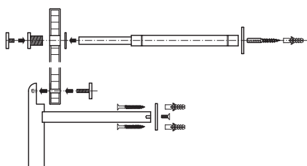
Montage mit Holzplatte
