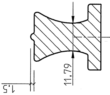
SEZIONE AA-AA
